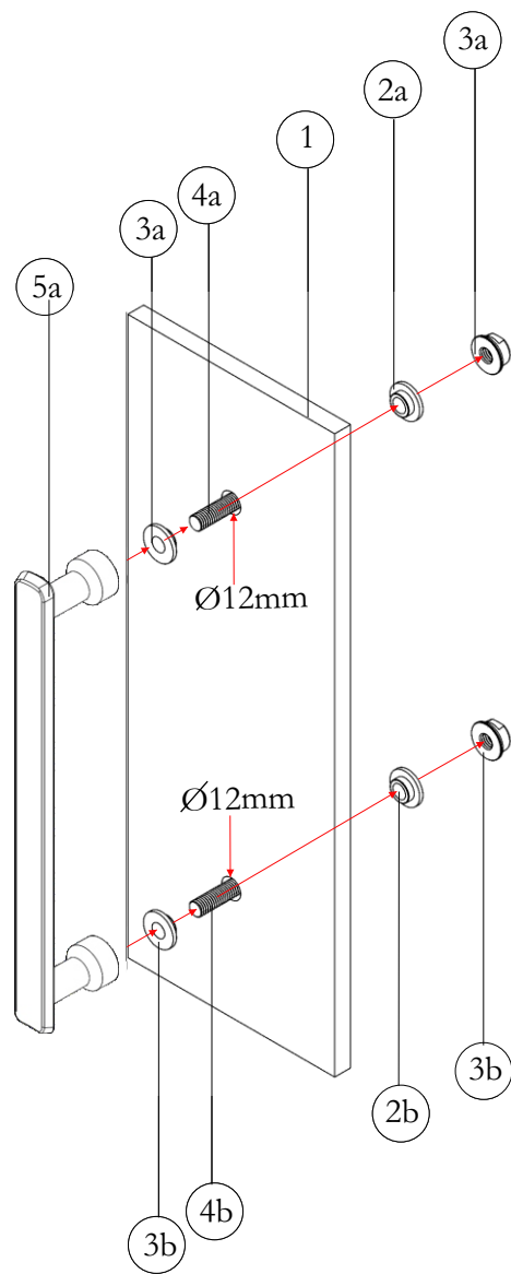
400-30-xx-01_300/S
